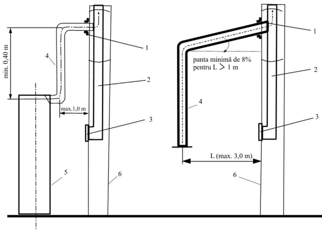
Fig. 13 Racordarea la coş de fum cu burlane
